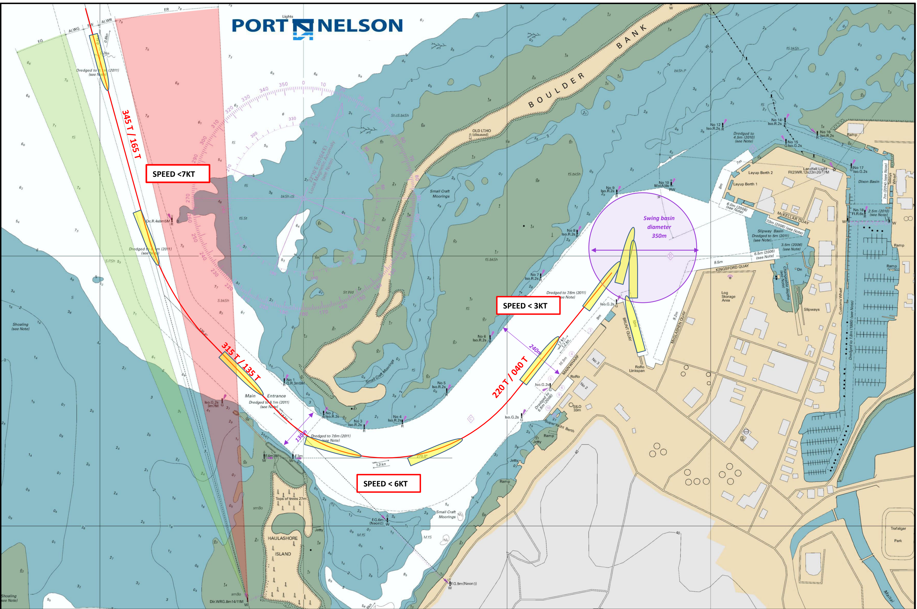
Manoeuvring Plan
